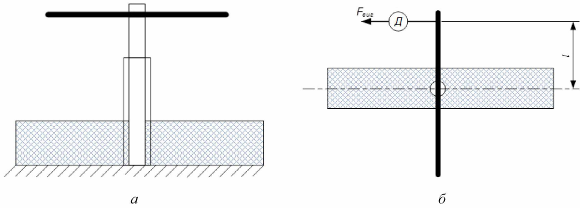
D – динамометр; F_{вит} – сила викручування; l – довжина важеля дії сили викручування.
